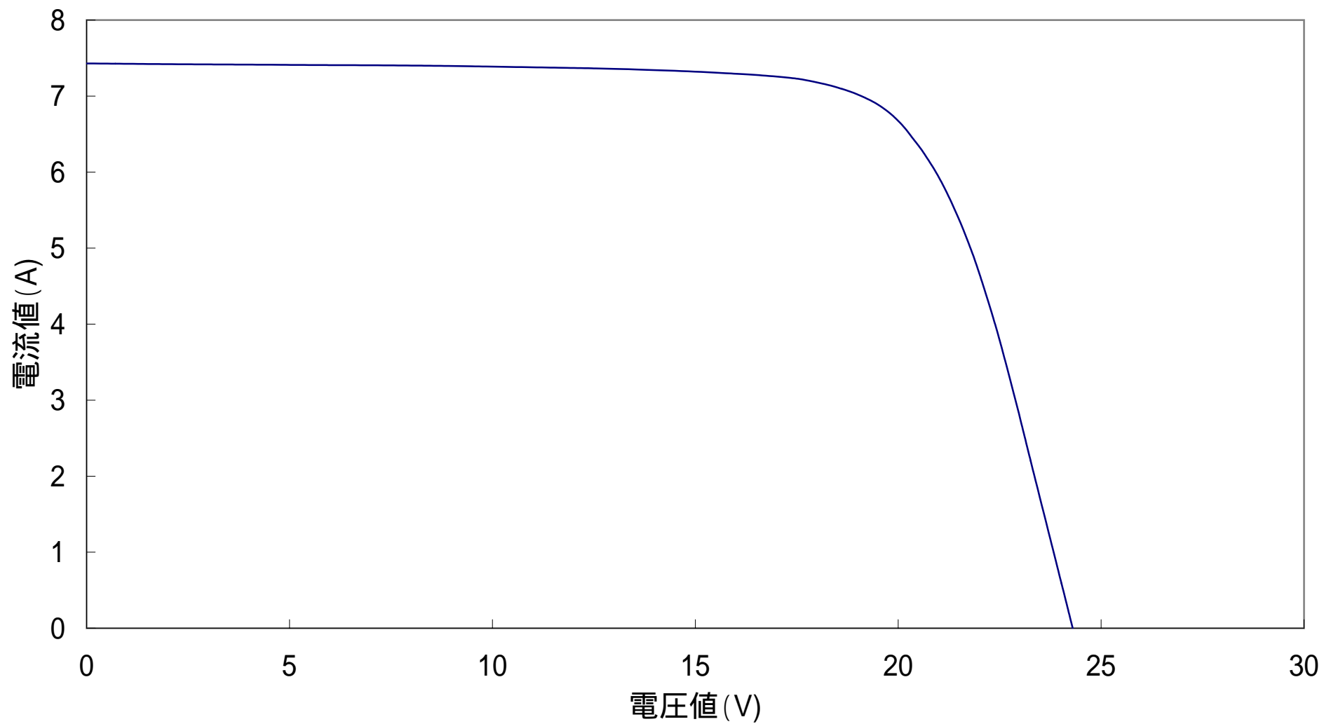
SJM134A-OBR 出力特性図 @1000W/m 2 AM1.5 25
